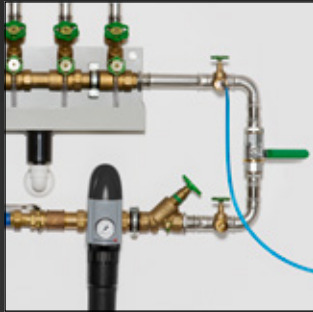
Druckprüfung mit Druckluft (SL/SLW) 4)7) Druckprüfung mit Wasser (SLW) 1)4)
